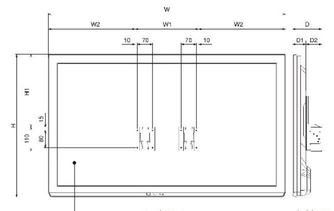
正視圖
